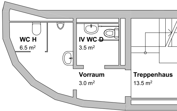
1. UNTERGESCHOSS
