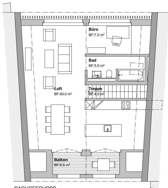
DACHGESCHOSS
