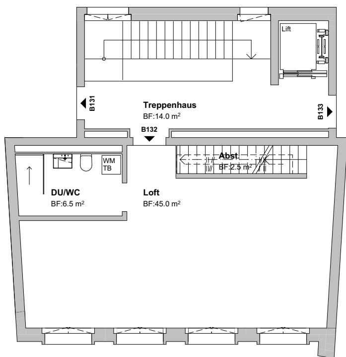
3.OBERGESCHOSS
